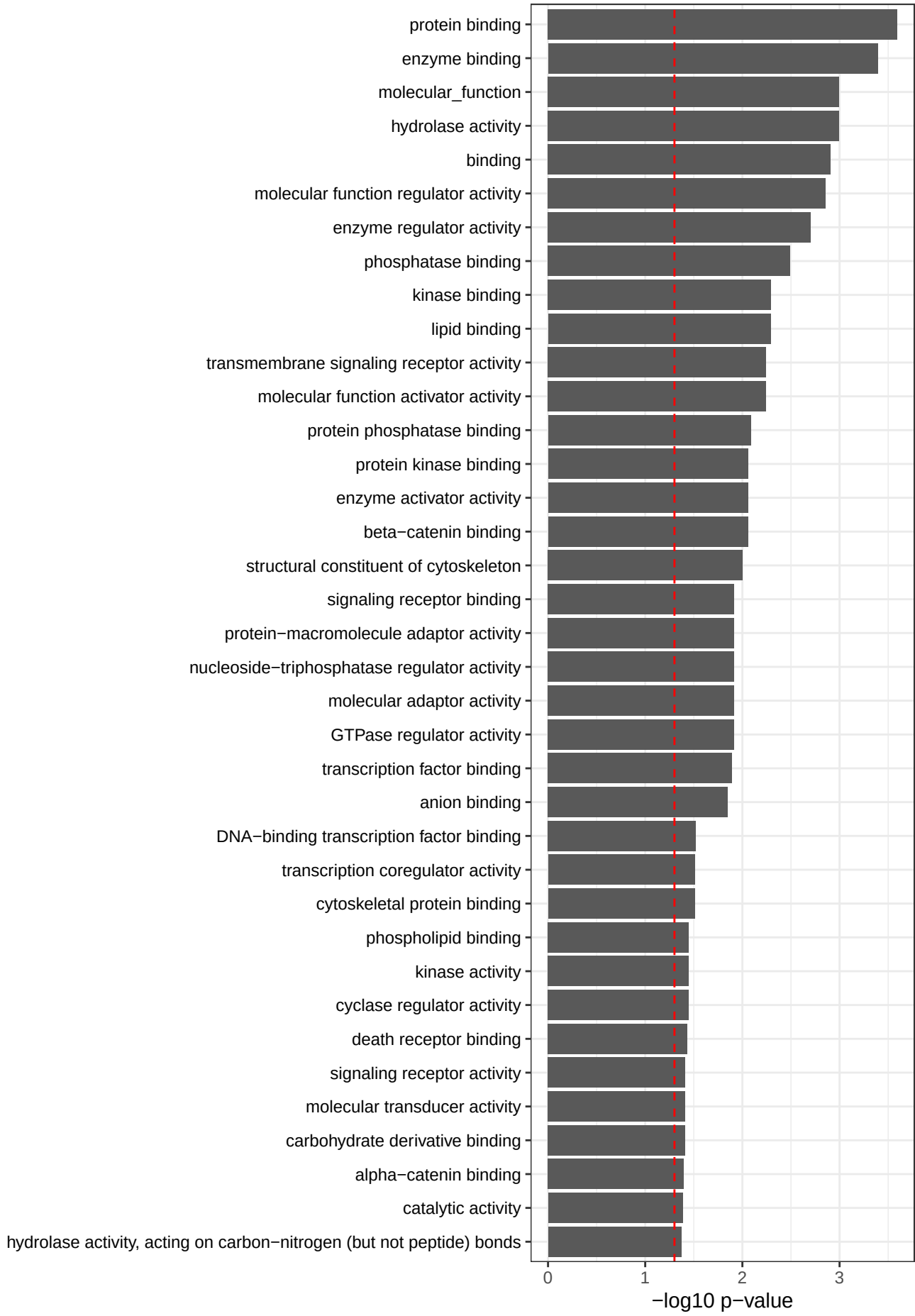
24 hour up DOX_DAR_DEG pairs (w
